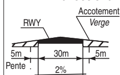
PROFIL EN TRAVERS DE LA PISTE RWY CROSS SECTION
